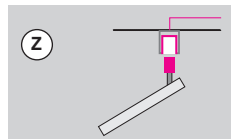
Montage mit Stromschienen-adapter für PALADIO TRACK System Installation with adapter for PALADIO TRACK system (48 V).
